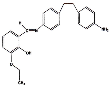
L 1 (E)-2-(((4(4-aminophenethyl)phenyl)imino)methyl)-6-ethoxyphenol
