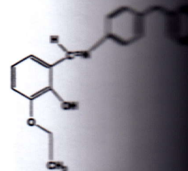
L 6 (E)-2-(((4-aminophenyl)imino)methyl)-6-ethoxyphenol
