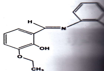
L 3 (E)-2-(((2-aminophenyl)imino)methyl)-6-ethoxyphenol
