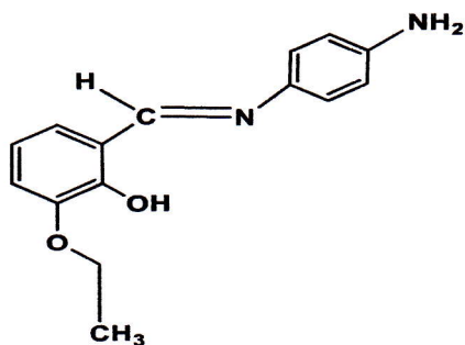
L 4 (E)-2-(((4-aminophenyl)imino)methyl)-6-ethoxyphenol
