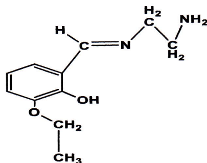
L 5 -(E)-2-(((2-aminoethyl)imino)methyl)-6-ethoxyphenol
