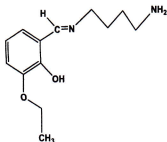
L 2 -(E)-2-(((4aminobutyl)imino)methyl)-6-ethoxyphenol
