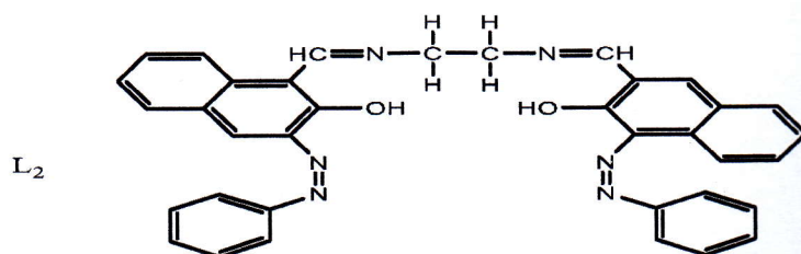
3-(((2-(((2-hydroxy-3-((Z)-phenyldiazenyl)naphthalen-1-yl)methylene)amino)ethyl)imino)methyl)-1-((Z)-phenyldiazenyl)naphthalen-2-ol
