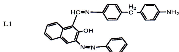
1-(((4-(4-aminobenzyl)phenyl)imino)methyl)-3-((Z)-phenyldiazenyl)naphthalen-2-ol
