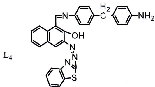
1-(((4-(4-aminobenzyl)phenyl)imino)methyl)-3-((Z)-benzo[d]thiazol-2-yl)diazenyl)naphthalen-2-ol
