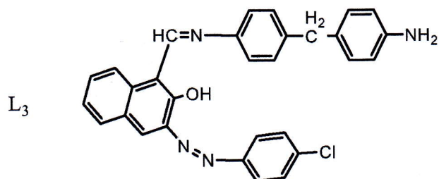
1-(((4-(4-aminobenzyl)phenyl)imino)methyl)-3-((Z)-(4-chlorophenyl)diazenyl)naphthalen-2-ol
